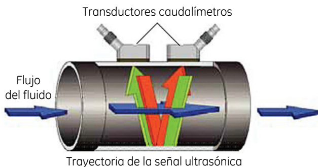
Técnica de medición de caudal por tiempo de tránsito
