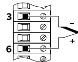
e - Thermocouple
