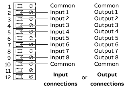
O7 Digital input / output module
