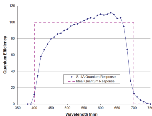
Plot A: PAR Smart Sensor Typical Quantum Response
