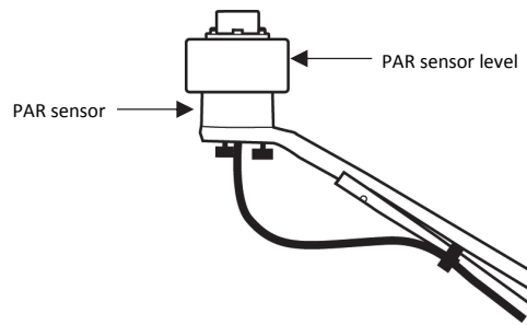
Leveling the PAR Smart Sensor on the Light Sensor Bracket
