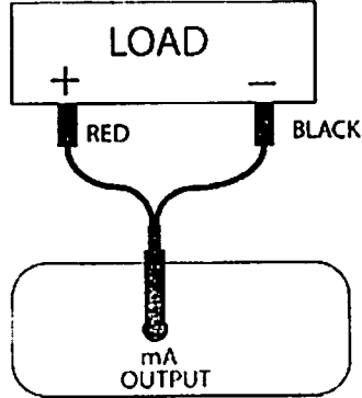
Fig. 2 mA Source Output
