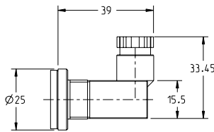
MICRO DIN (9.4 mm)
