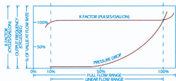
Typical K-Factor Curve (Pulses per Gallon)
